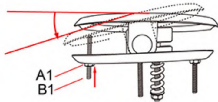
Dra åt B1-skruven uppåt och dra åt A1-muttern
