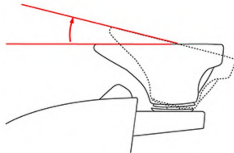
Justera lutningsvinkeln för det keramiska handfatet nedåt
