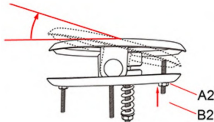
Dra åt B2-skruven uppåt och dra åt A2-muttern
